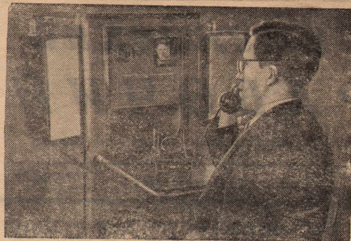
Ленинград. Старший научный сотрудник Всесоюзного научно-исследовательского института телевизионной техники И. П. Захаров разработал схему и изготовил малогабаритную телевизионную камеру, позволяющую во время телефонного разговора видеть собеседника. Первые опытные видеотелефоны установлены в институте. На снимке: И. П. Захаров у видеотелефона. Фото Н. Янова. Прессклише ТАСС.
