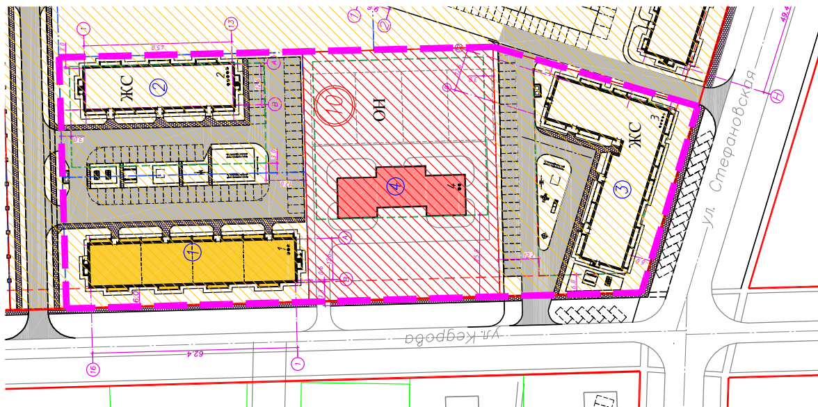
Чертёж планировки территории. (Основной чертёж с эскизом застройки М 1:2000)
